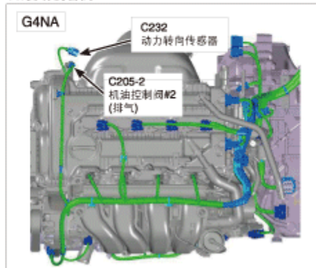
44.发动机右侧
