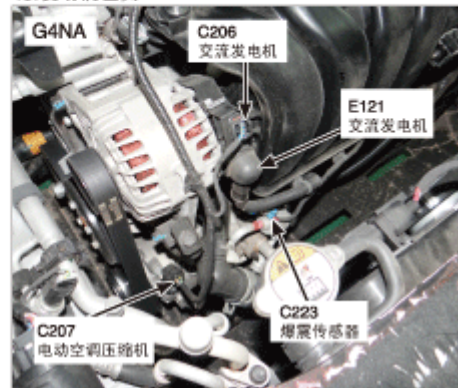
45.发动机左侧
