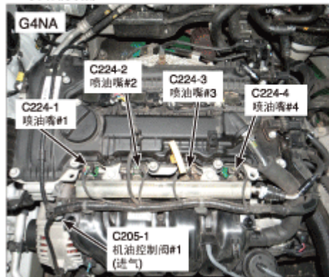
43.发动机顶部
