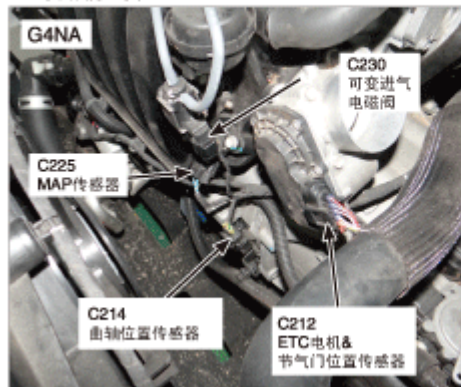
46.发动机左侧
