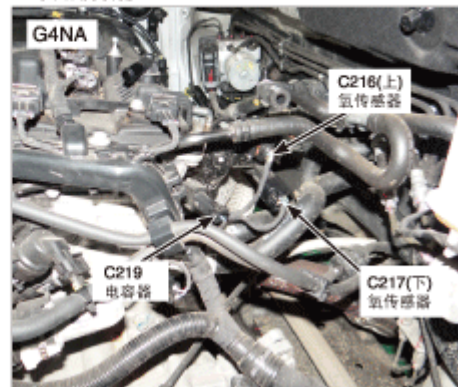
48.发动机后部
